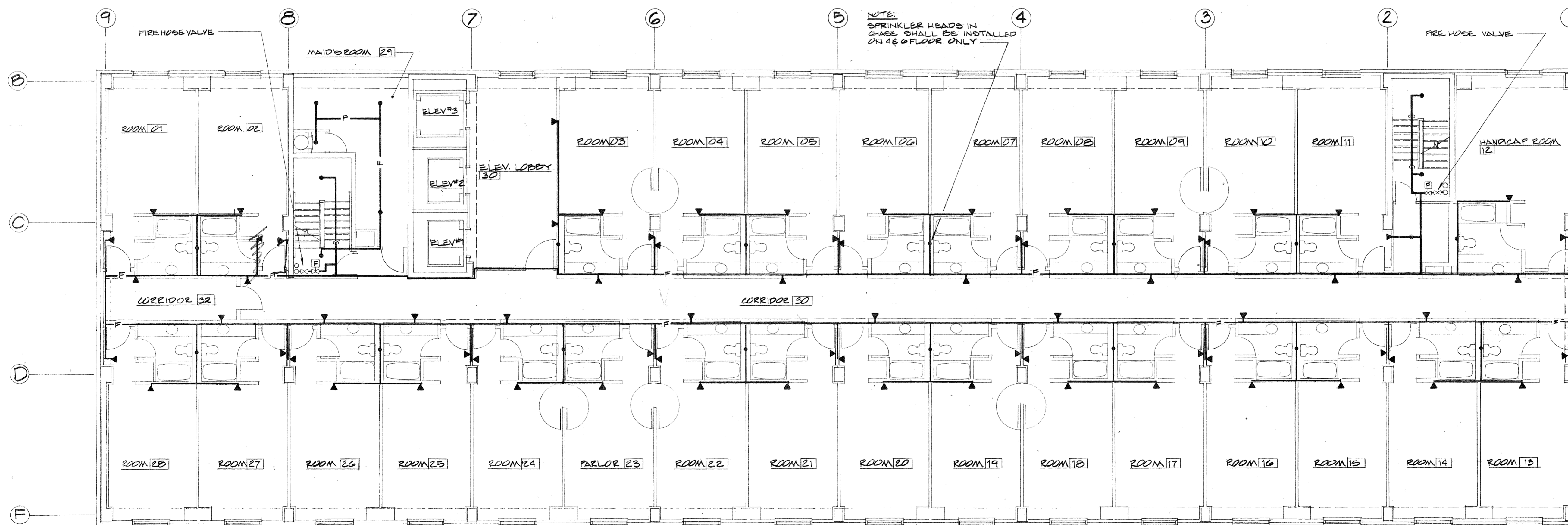
SPRINKLER PLAN - 3 RD THRU 7 TH FLOORS SCALE: 1/8" = 1'-0"
